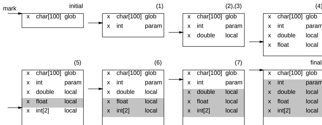
図 2: 線形探索で実現した記号表
