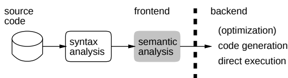
図 1: 意味解析の位置づけ
