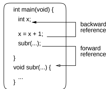
図 4: 前方参照・後方参照
