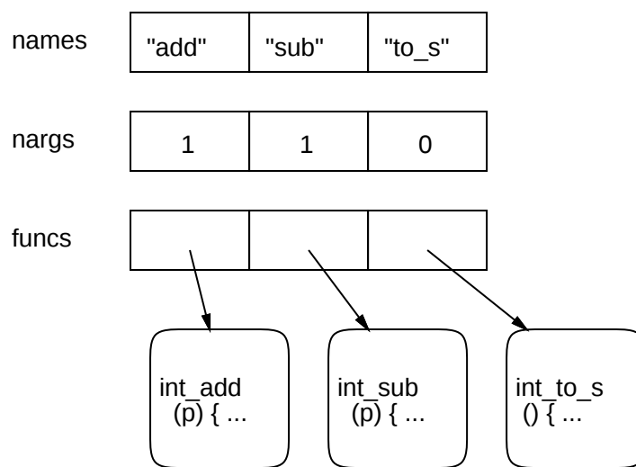
図 1: メソッドテーブルの実装例
