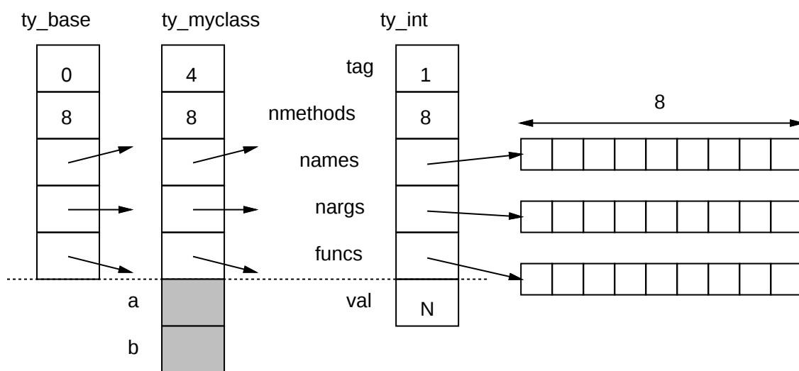
図 2: オブジェクトの構造
