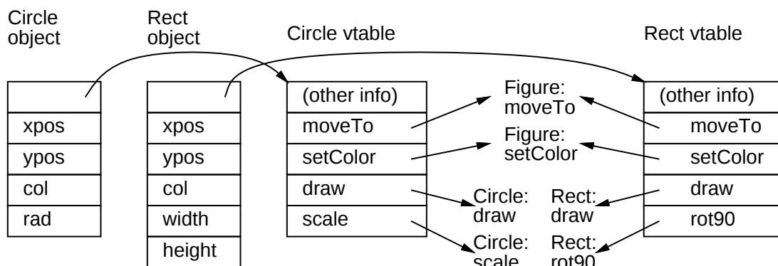
図 3: 単一継承向けの静的な配置
