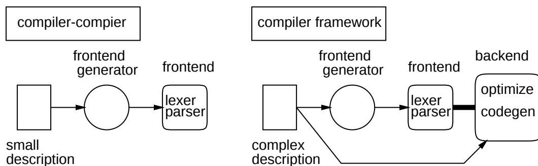
図 1: コンパイラコンパイラ の概念
