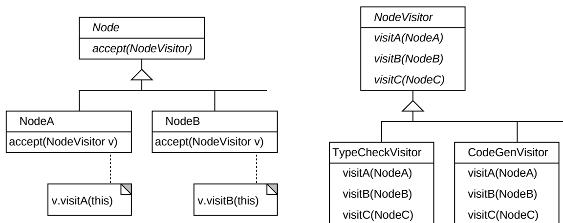
図 3: Visitor パターンへの変換
