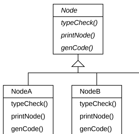
図 2: 素朴な再帰による木構造の処理
