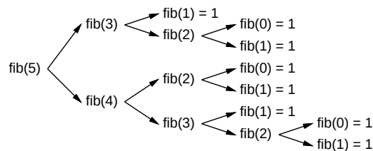
図 1: fib 再帰関数での計算の重複
