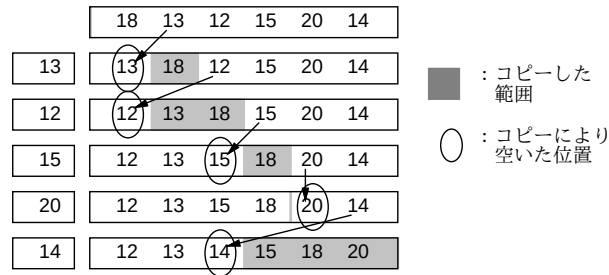
図 4: 単純挿入法
