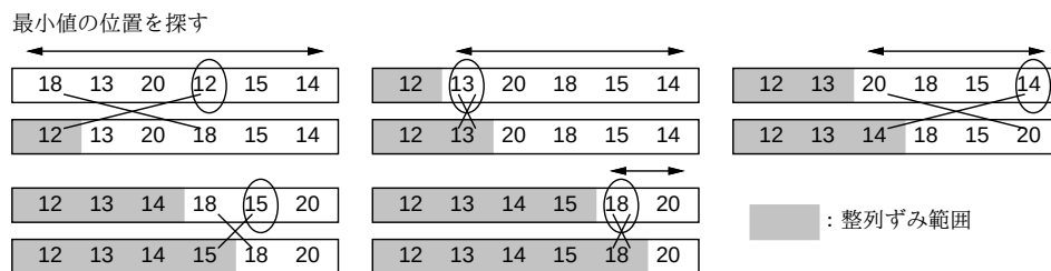
図 3: 単純選択法
