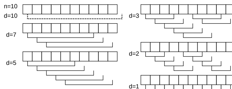
図 6: コムソート
