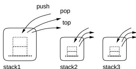
図 1: 抽象データ型としてのスタック
