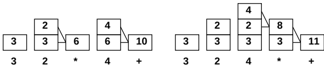
図 6: スタックを用いた後置記法の計算
