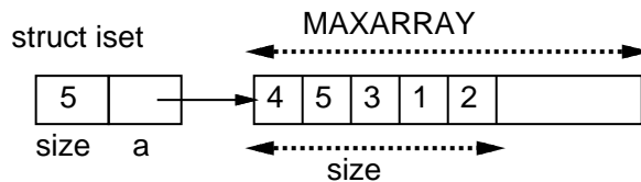
図 2: 整数の集合の実装
