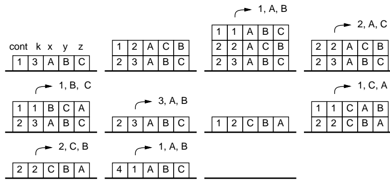
図 3: ハノイの塔のスタック版でのスタックの動作
